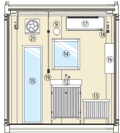
左側面図
